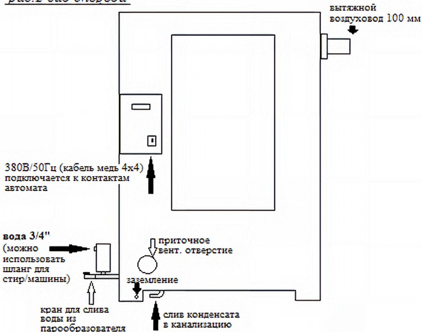
рис.2 вид спереди
